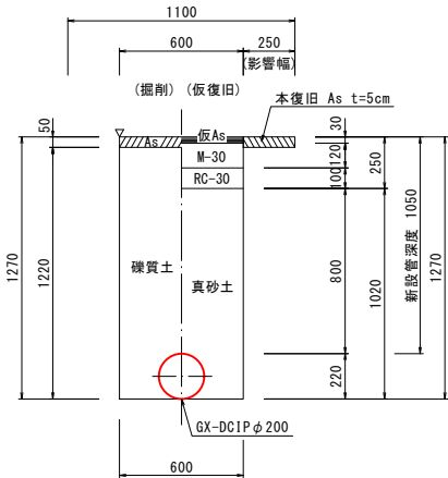
配管布設土工 ②
