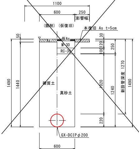
配管布設土工 ③
