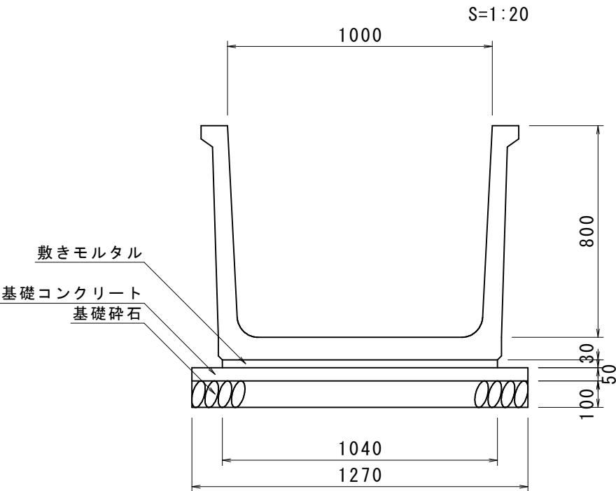
大型フリュームB1000×H800
