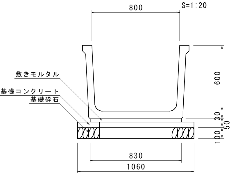
大型フリュームB800×H600
